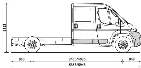
Châssis Double Cabine
