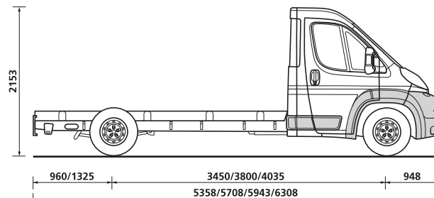
Châssis Cabine Version 4T
