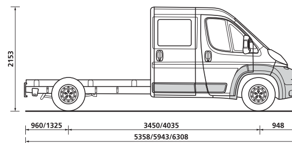
Châssis Double Cabine Version 4T
